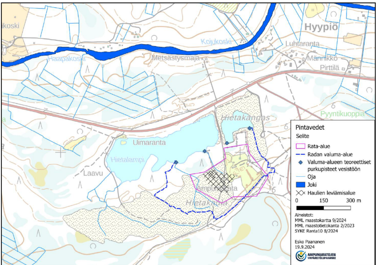
Kuva 6. Ampumarata-alueen valuma-alueetarkastelu.
