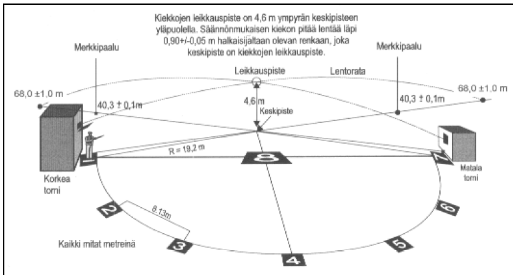
Kuva 11. Kuvakaavio skeet-radasta. (Suomen Ampumaurheiluliitto, 2015)
